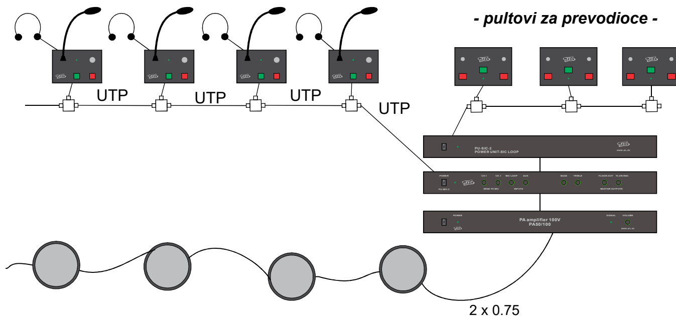
Blok šema vezivanja mikrofona i pulteva
